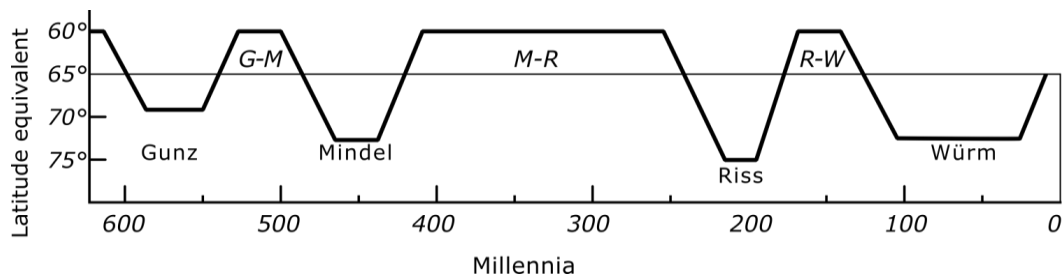
Figure 7: Penck and Brückner's scheme of glacial/interglacial periods in the Alps. Reprinted from Kanon der Erdbestrahlung und seine Anwendung auf das Eiszeitenproblem (p.417) by Milankovitch, M., 1941, Belgrade: Royal Serbian Academy Special Publications.
